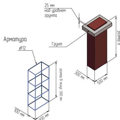
Фундамент опорной рамки
