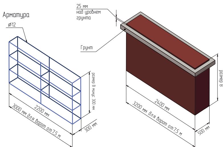
Фундамент рамки ворот
